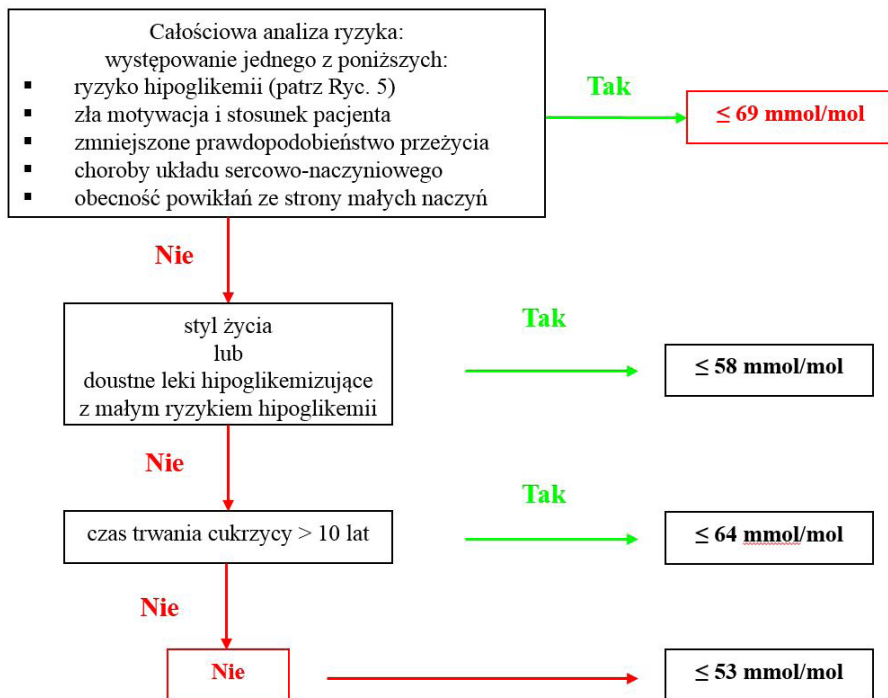
Rycina 3 (Oryg. 4) Algorytm osiągania wartości docelowych HbA1c u pacjentów z cukrzycą i CKD w stadium 3b lub wyższym (eGFR <45 mL/min).
